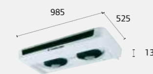
ÉVAPORATEUR ULTRAPLAT ES200
